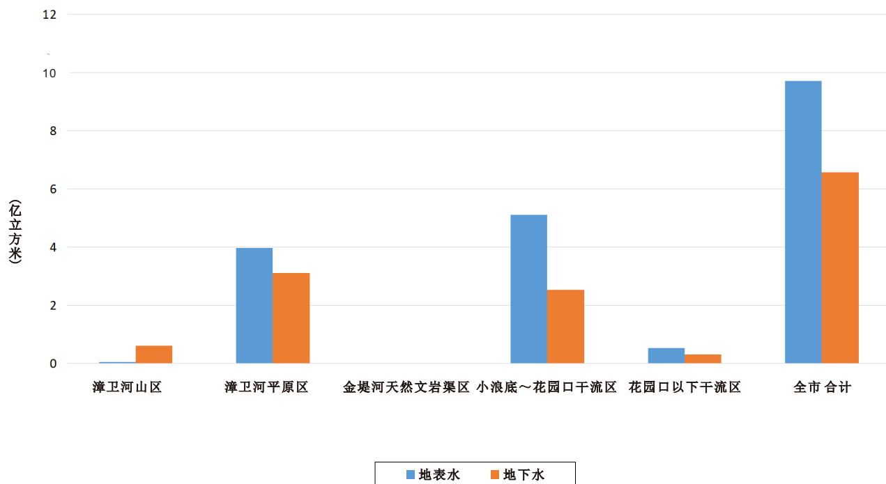
图六 新乡市水资源分区供水量组成图
