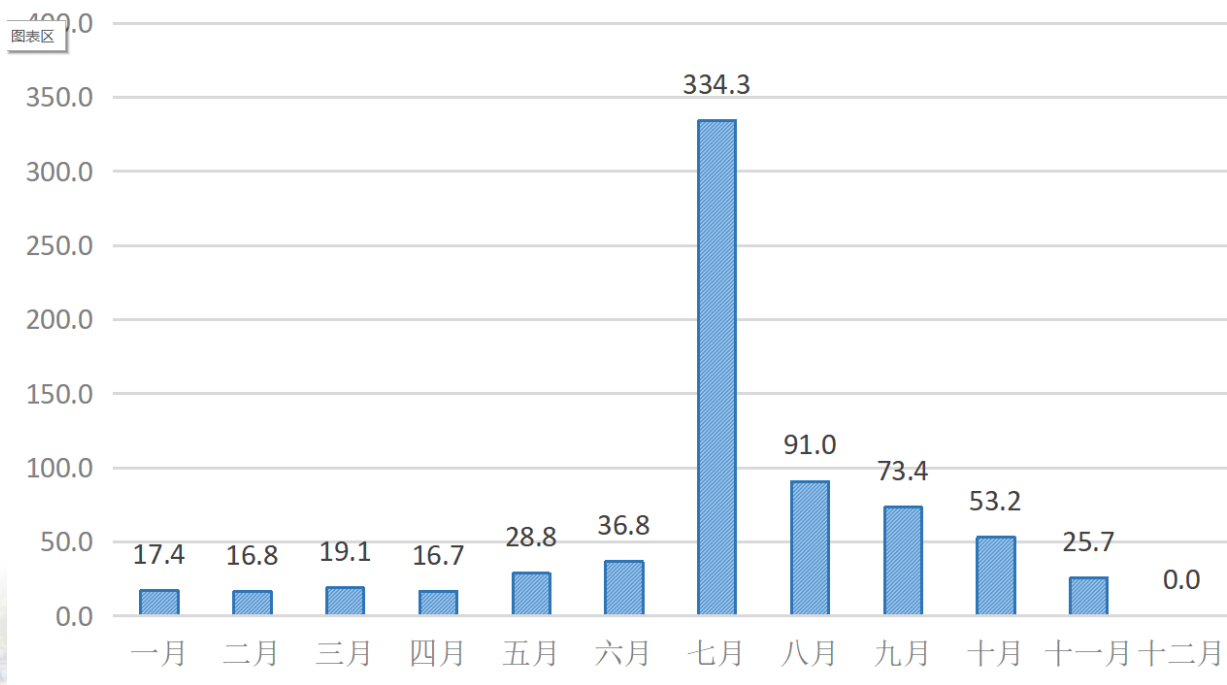
图二 新乡市降雨量分布图
