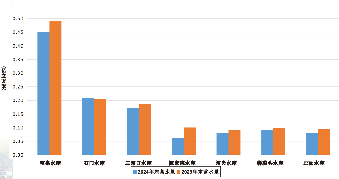
图四 新乡市水库蓄变量对比图
